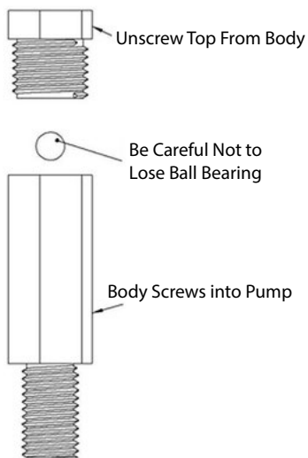
Rotorflush Air Bleed Valve
